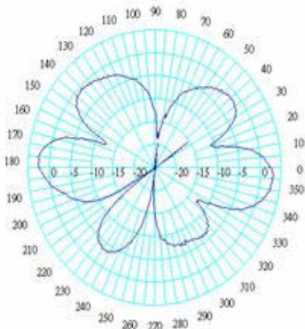
E-Plane
