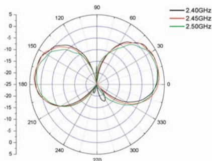
E-Plane (2.4 GHz—2.5 GHz)
