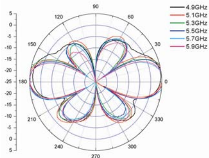
E-Plane (4.9 GHz—5.875 GHz)
